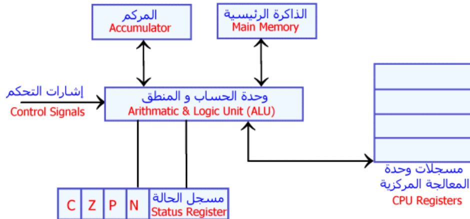
الشكل 8-1 وحدة الحساب والمنطق
