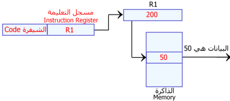
الشكل 1-19 العنونة غير المباشرة باستخدام مسجلات وحدة التحكم
