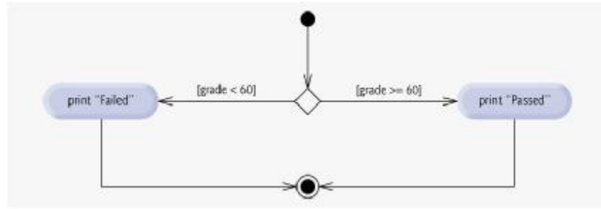
الشكل 5-2 المخطط الصندوقي لبنية if/else
