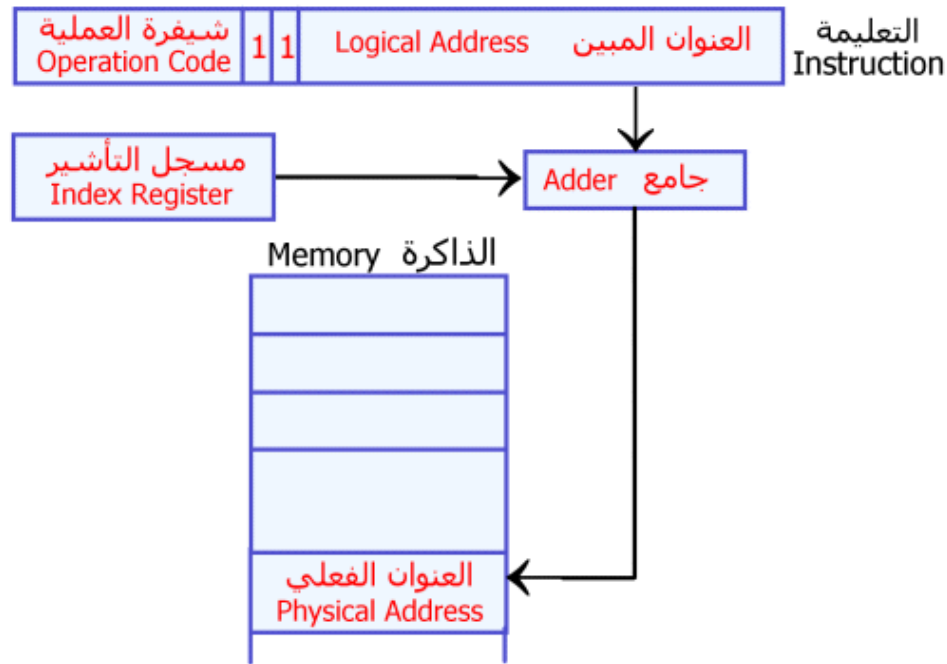
الشكل 1-21 طريقة الحصول على العنوان الفعلي في العنونة غير المباشرة - المؤشرة
