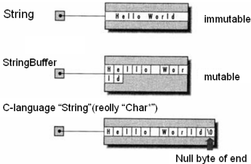
الشكل 8-1 رسم توضيحي لبنية كل من الصنف String والصنف StringBuffer
