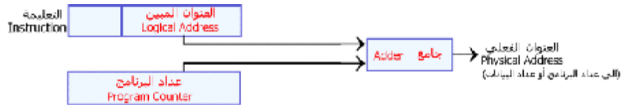
الشكل 1-22 طريقة الحصول على العنوان الفعلي في العنونة النسبية
